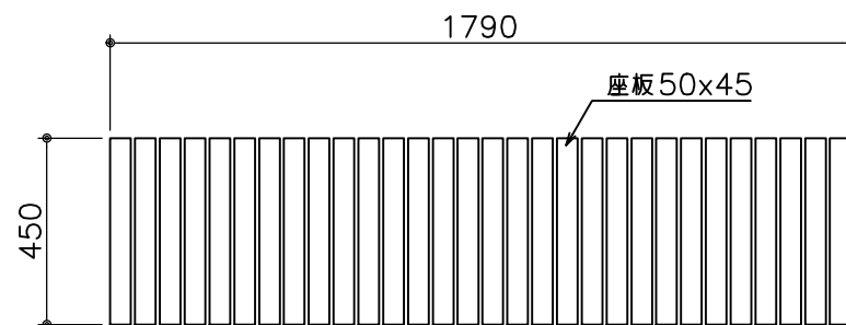
平面図 S=1:20
