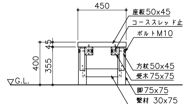
断面図 S=1:20
