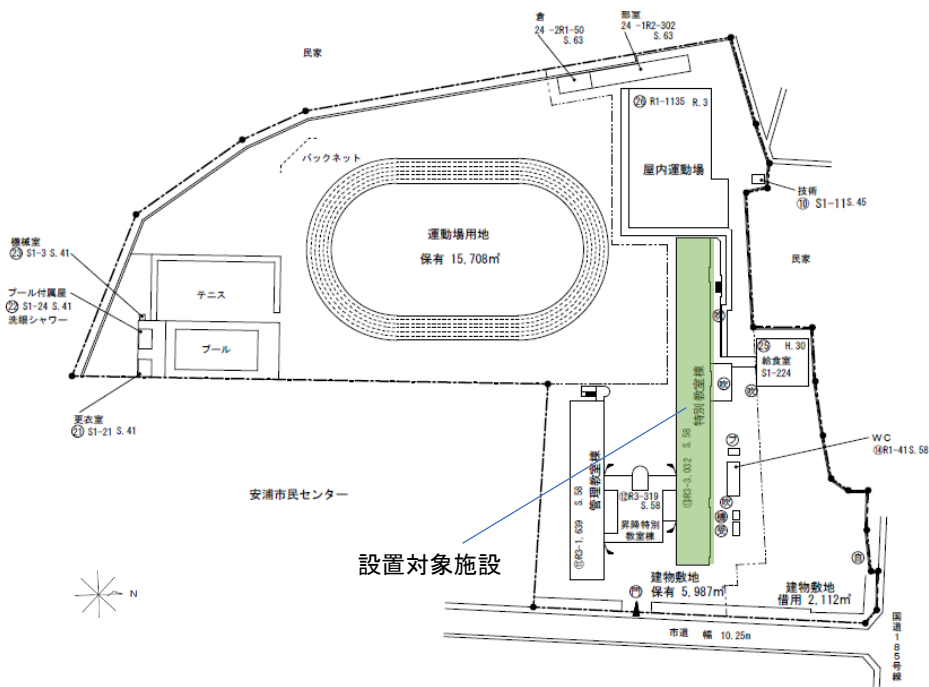
第 1 図 安浦中学校施設配置図 (S=NON)
