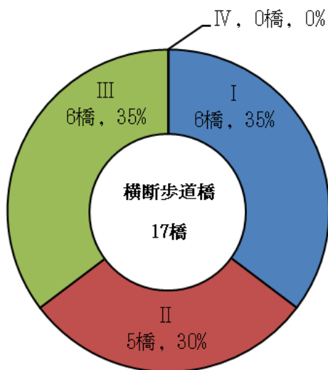
図 5-1 定期点検結果に基づく健全性
