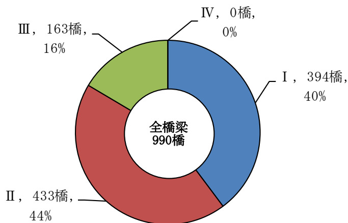
図 5-1 定期点検結果に基づく健全性
