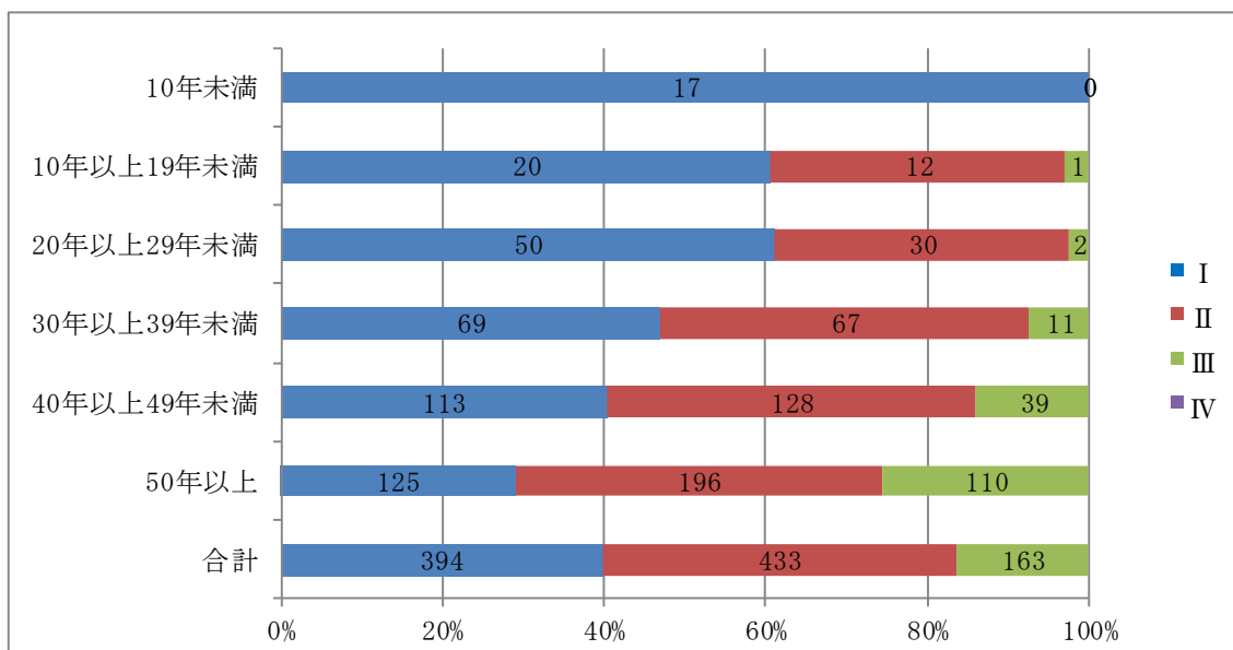
図 5-2 判定区分と建設経過年数
