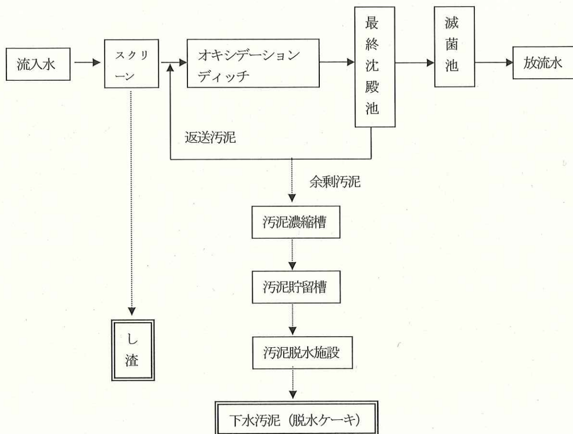
図1 安浦浄化センターでの工程
