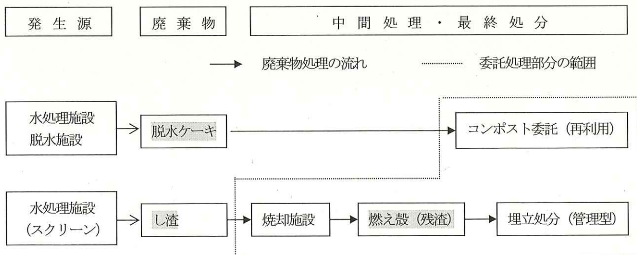
図2 処理の工程
