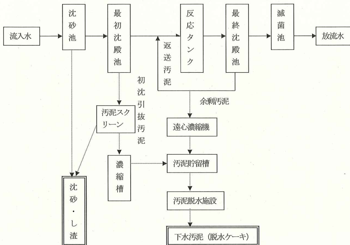
図1 広浄化センターでの工程
