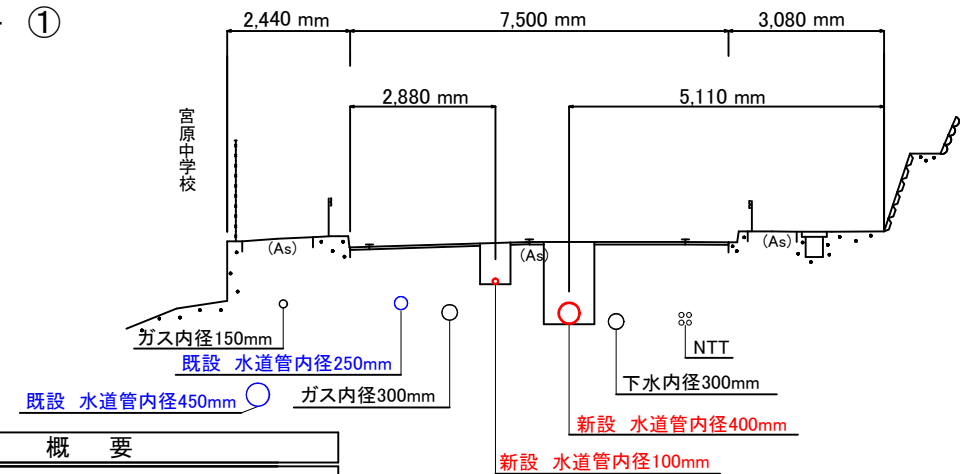
横断面図 S=1:150
