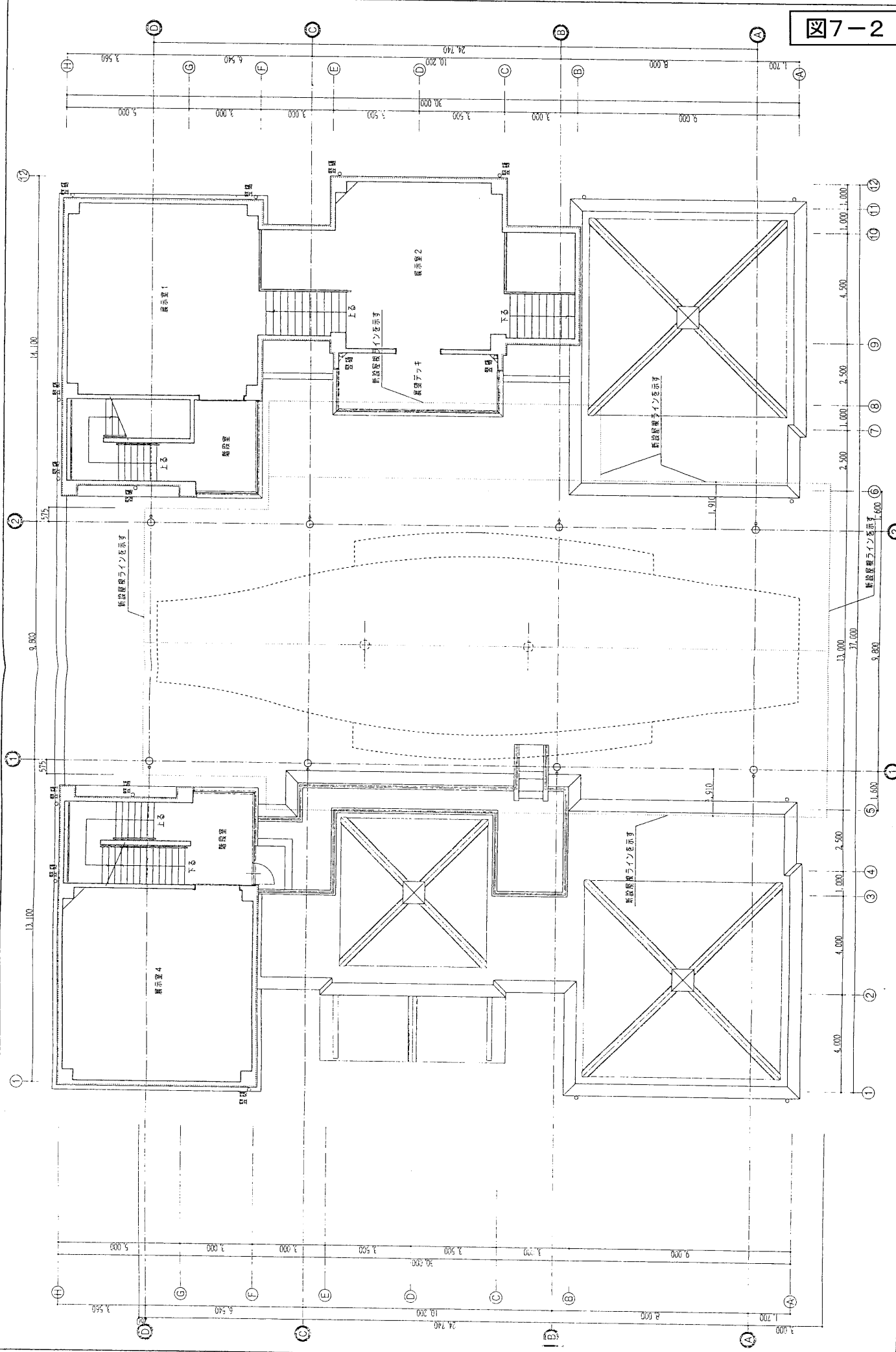
長門の造船歴史館 2階
