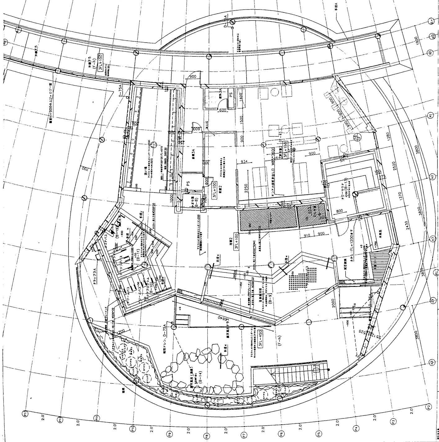
くらはし桂浜温泉館平面図 A棟3階
