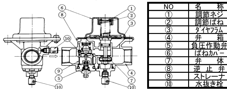
減 圧 弁
