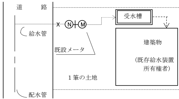
例（分割後） 図-2-3-4-（2）
