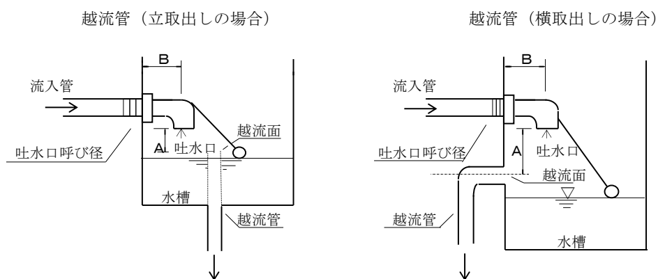
図-9-1-8 吐水口空間標準図
