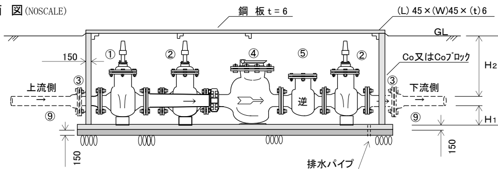
側 面 図 (NOSCALE)
