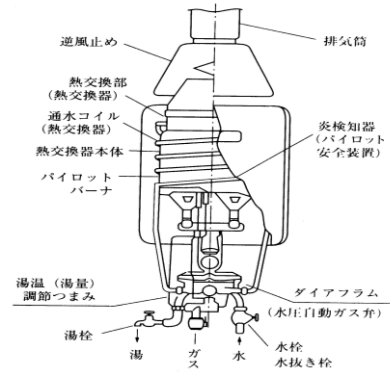
瞬間湯沸器(先止め式)
