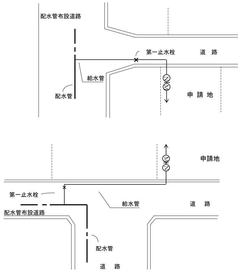
配水管の布設していない道路を通過するときの例
