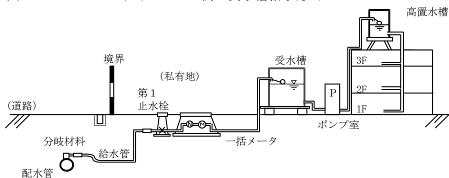
図-2-3-10-(1) 例 受水槽給水方式
