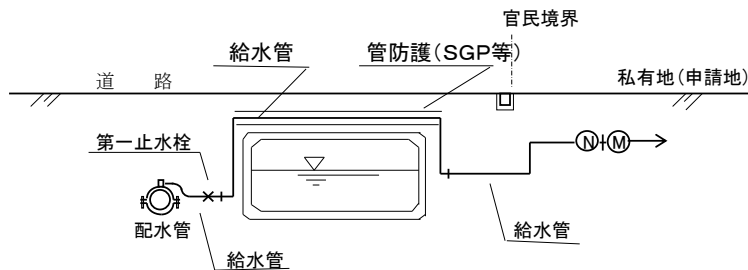
上越配管の例
