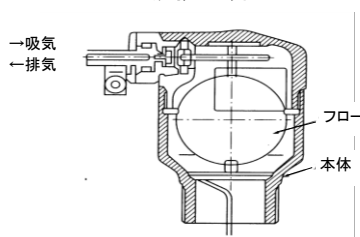
吸排気弁
