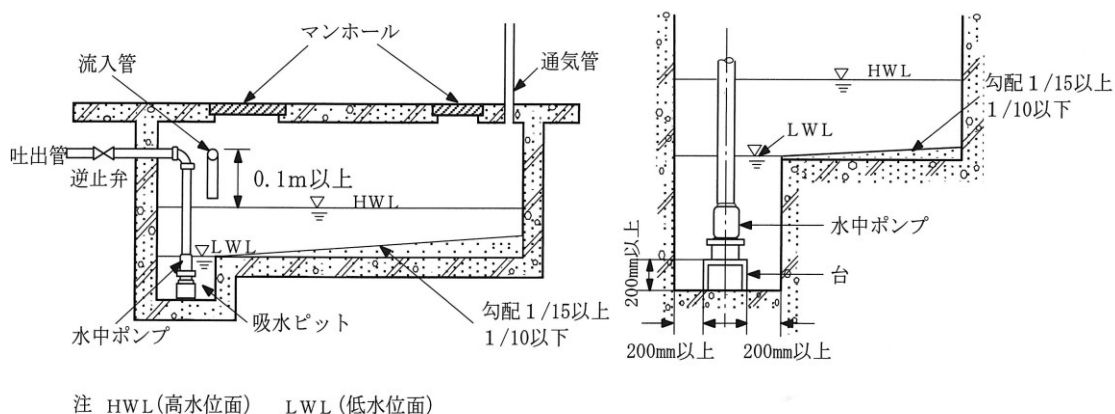
図4-15 排水槽の例
