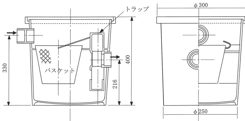
図4-23 分離ますの例
