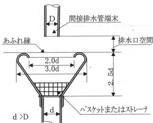
図 4 - 1 7 排水口空間
