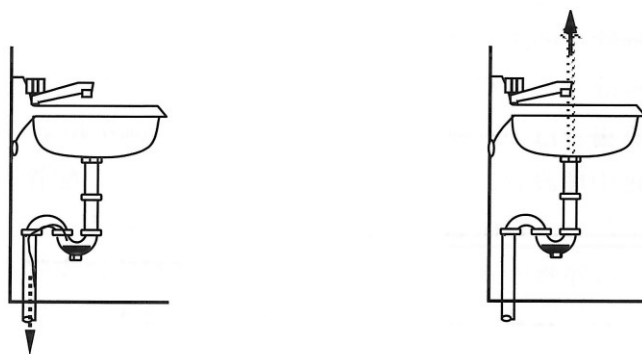
図4-6 毛管現象
