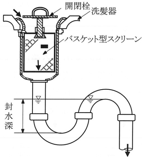
図 4-12 ヘア阻集器の例
