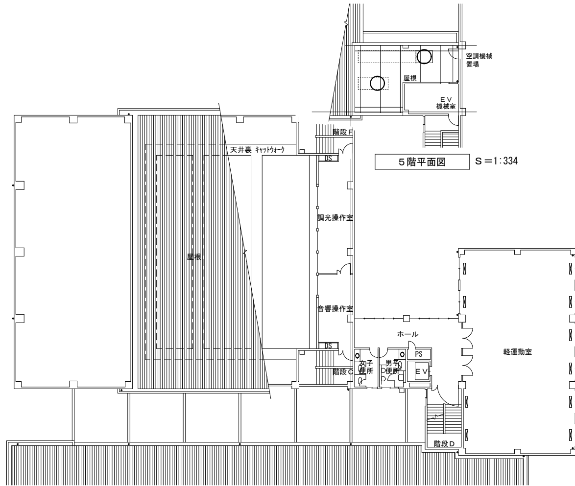
4階平面図 S=1:334
