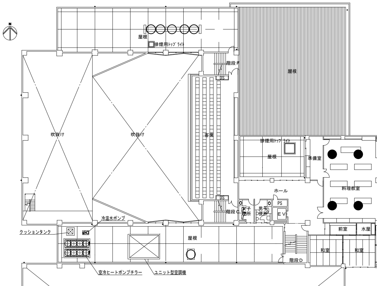
3階平面図 S=1:334
