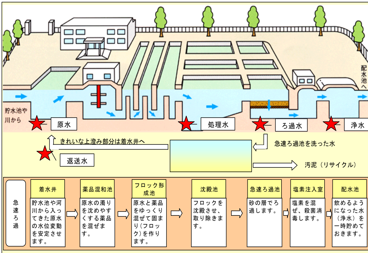
(図4) 浄水場の概略図と検査地点
