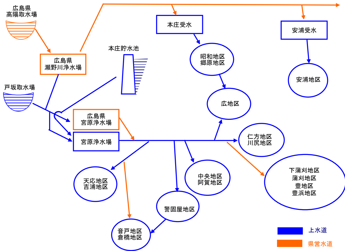
(図1) 配水系統図
