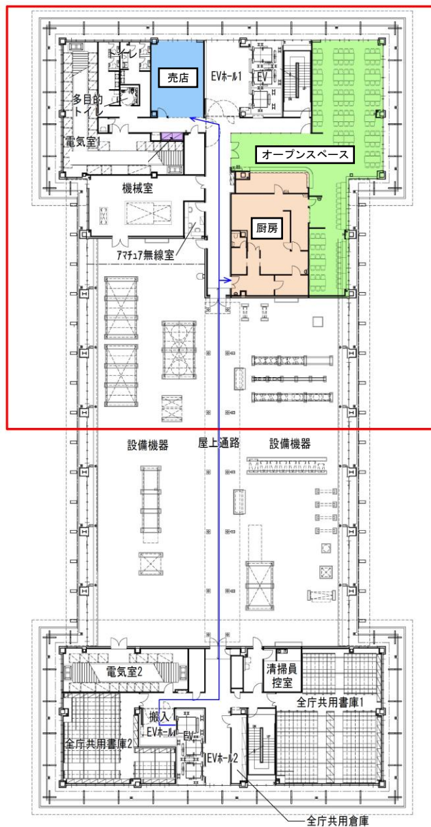
平面図 (9階)
