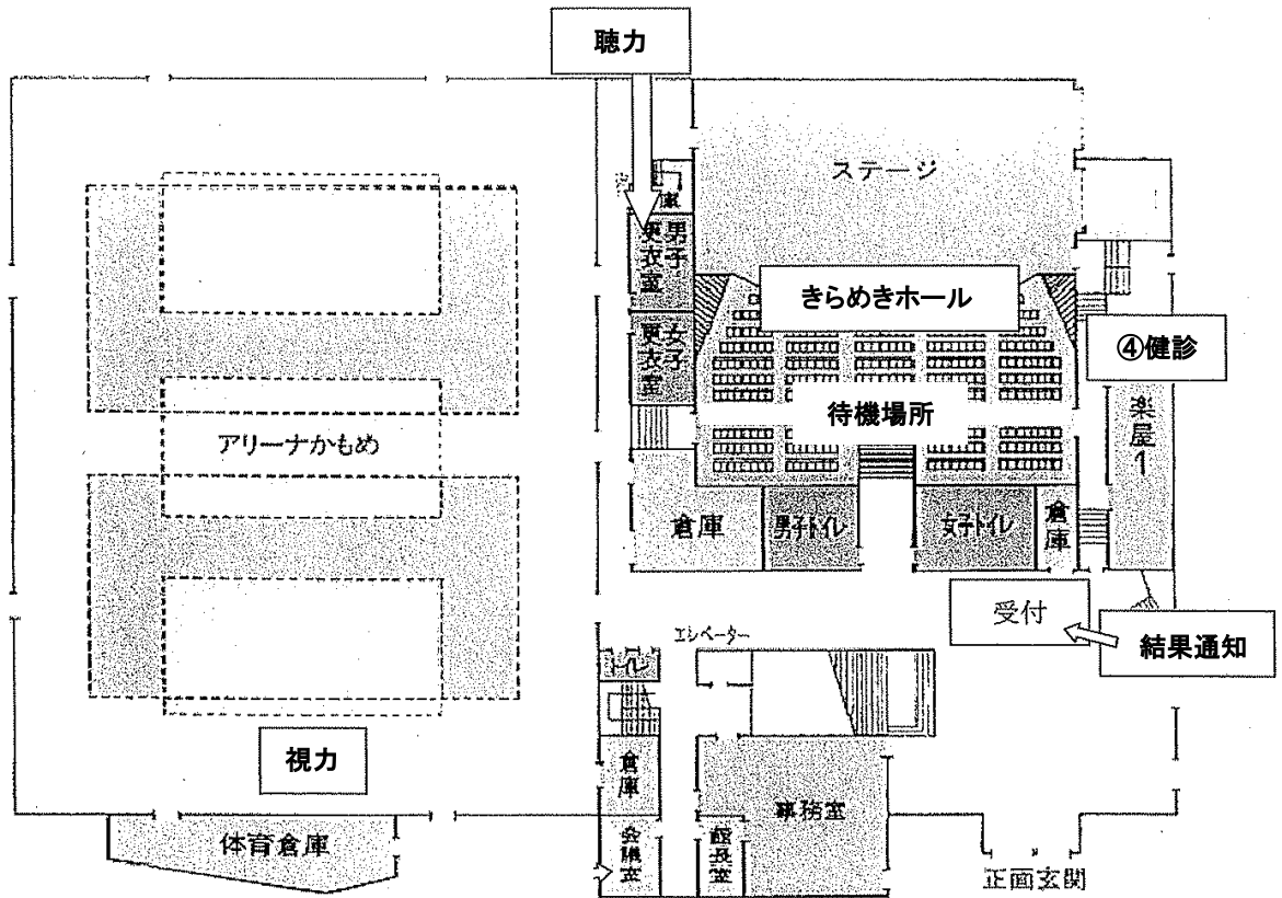
館内1F平面図
