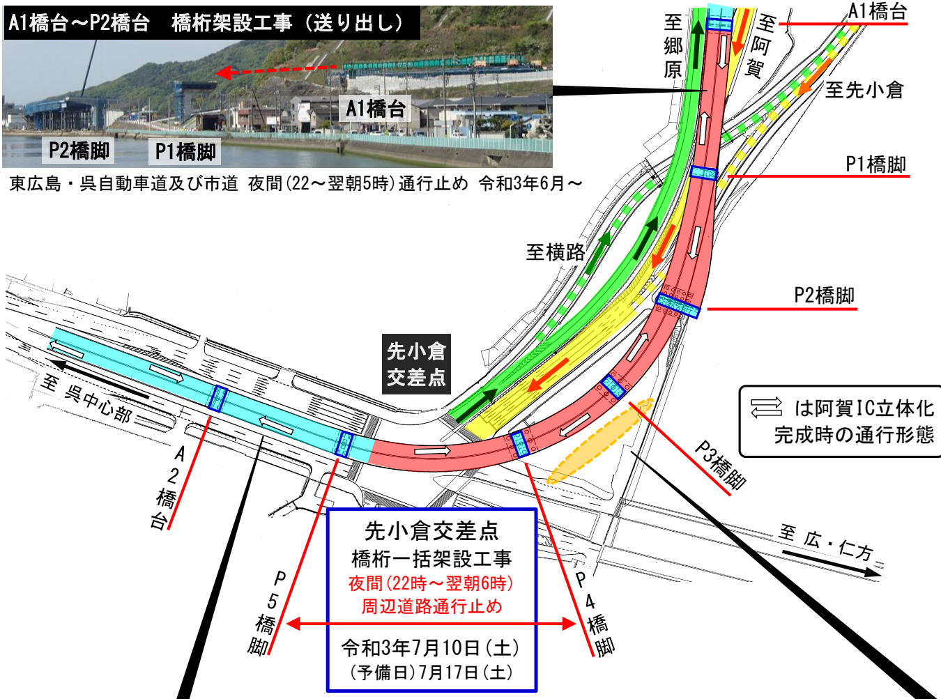
橋桁架設(A2橋台～P5橋脚間)
