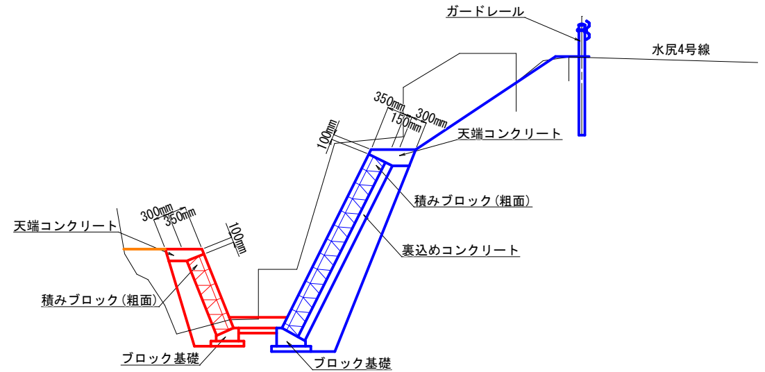
コンクリートブロック積み
