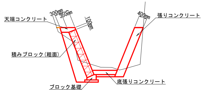
コンクリートブロック積み
