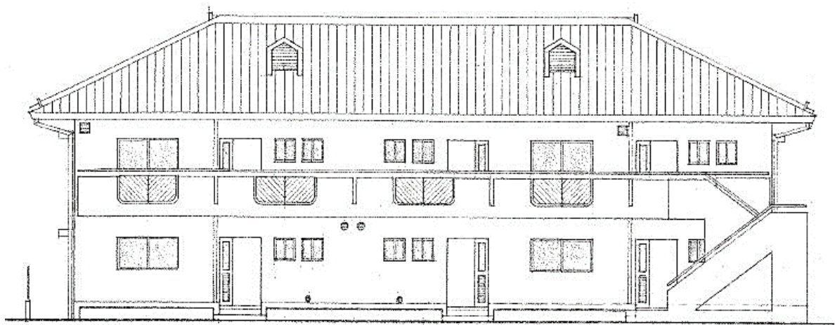
建物立面図
