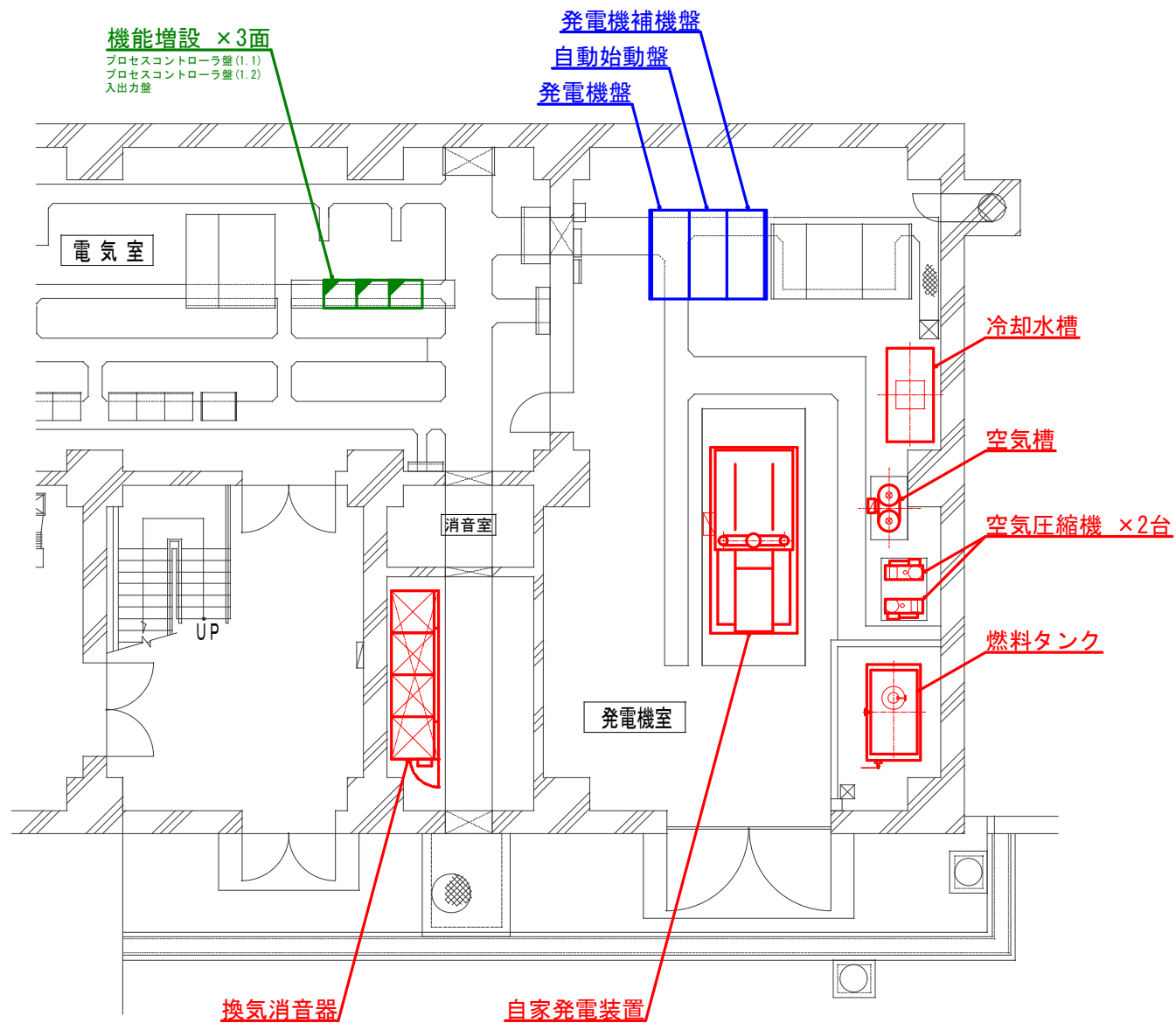
活性炭注入棟 1階 平面図
