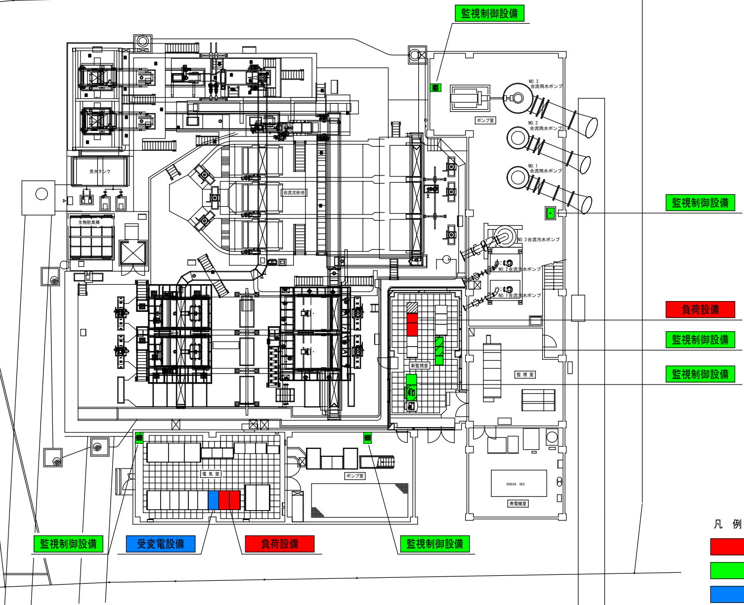
二河川ポンプ場全体平面図 1/280
