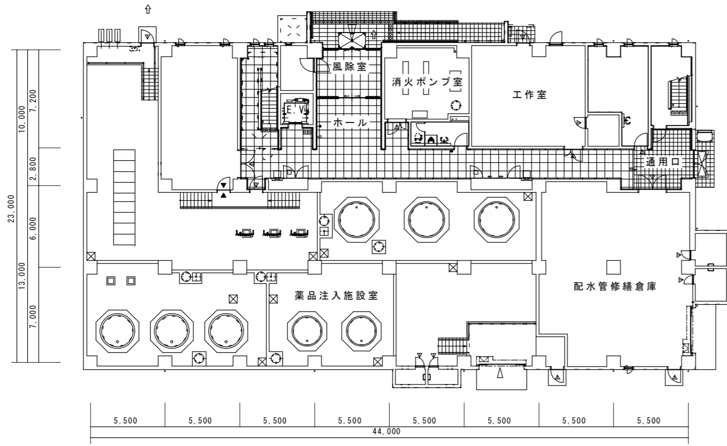
1階平面図
