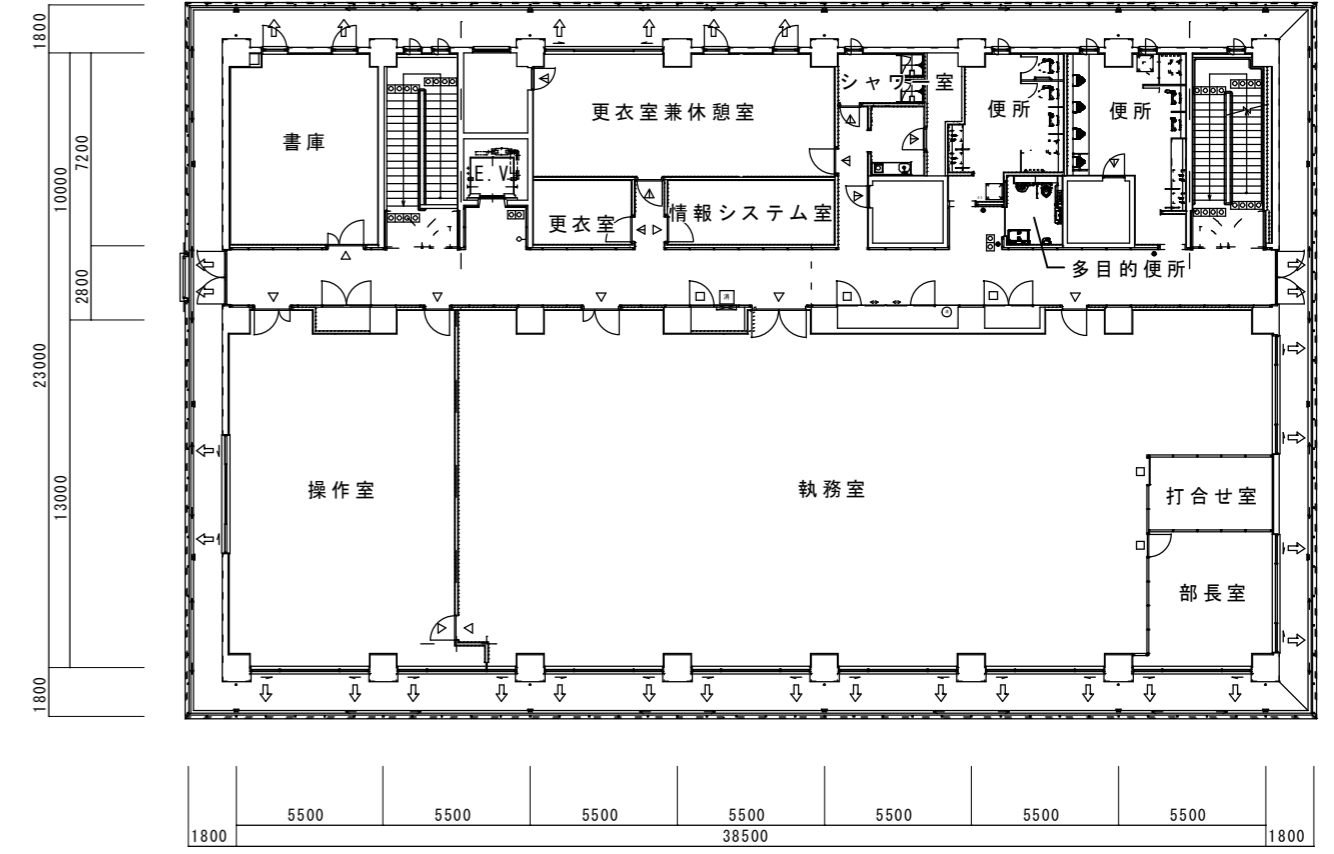
3階平面図
