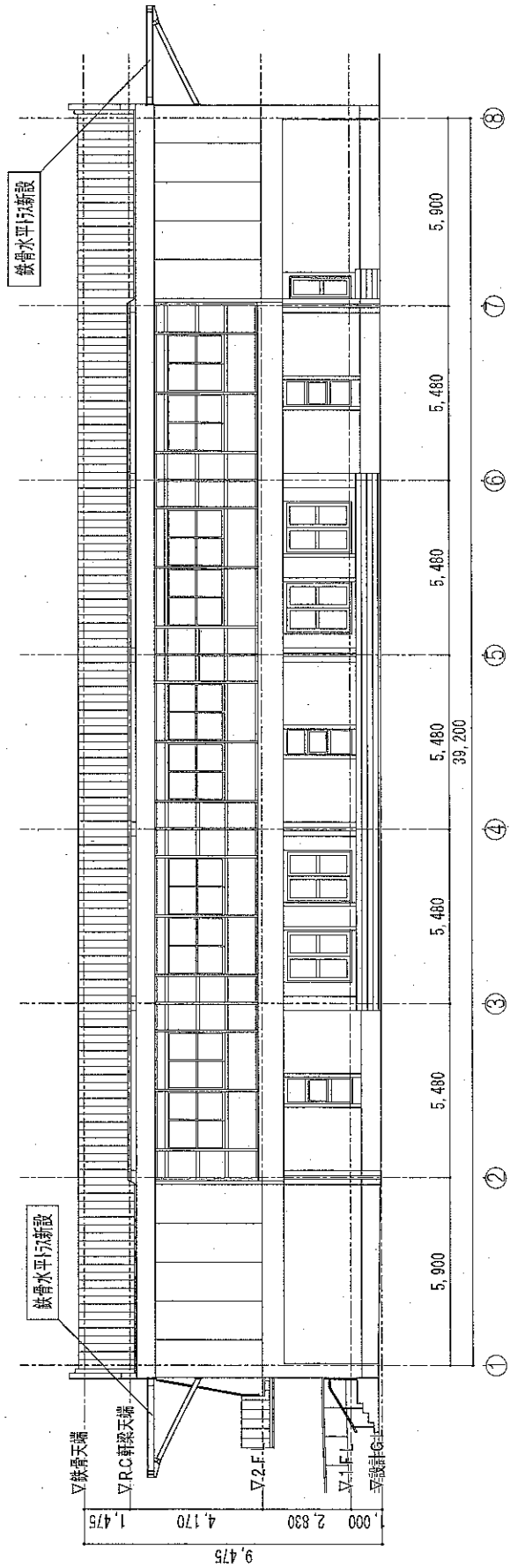
多目的ホール 東立面图 1/200
