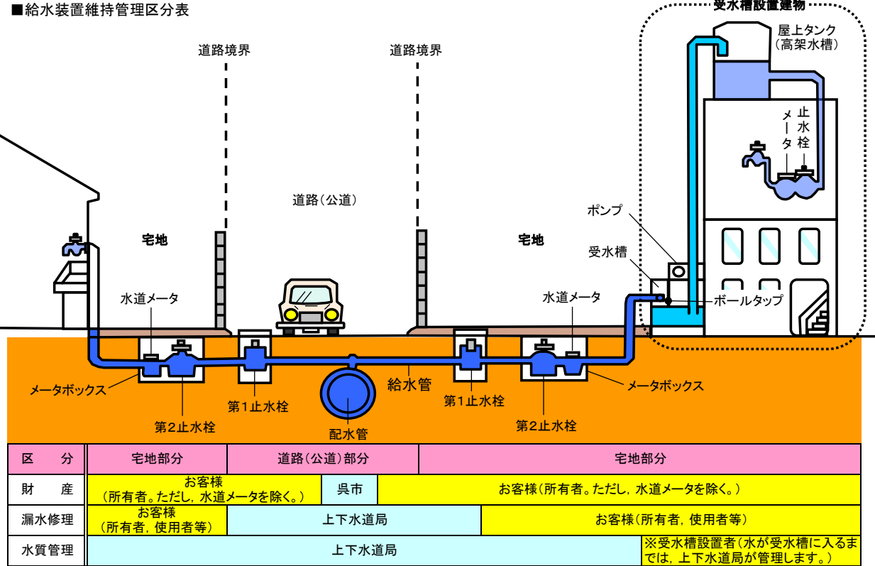
■給水装置維持管理区分表
