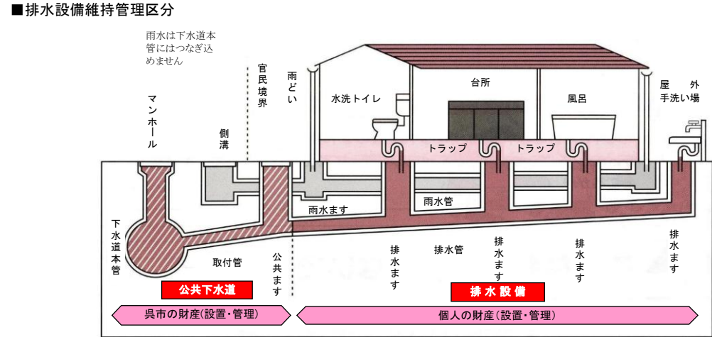
■排水設備維持管理区分
