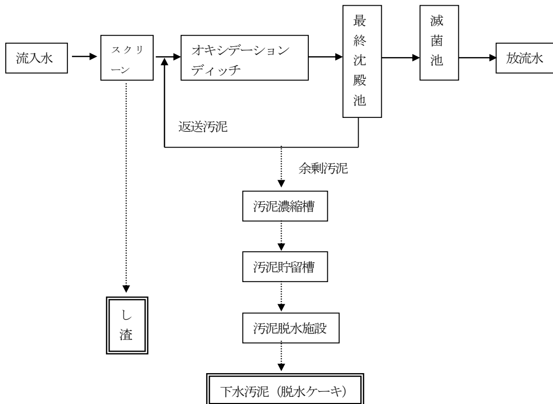
図1 安浦浄化センターでの工程
