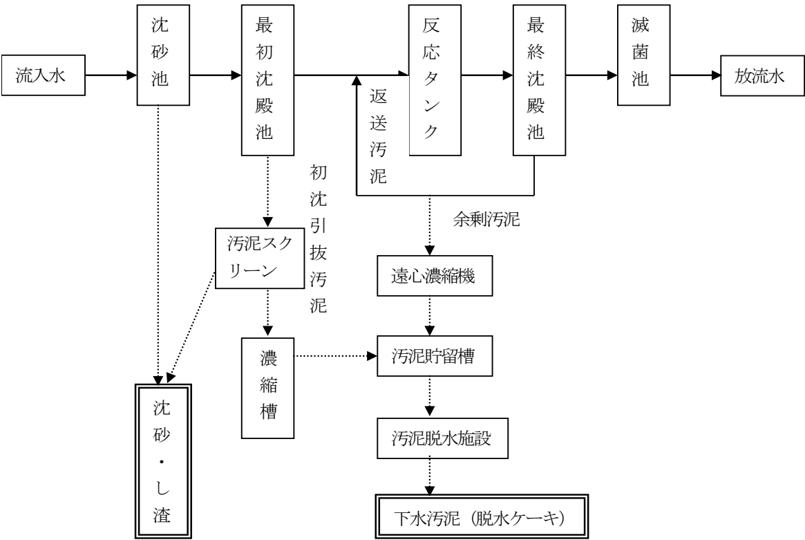
図1 広浄化センターでの工程
