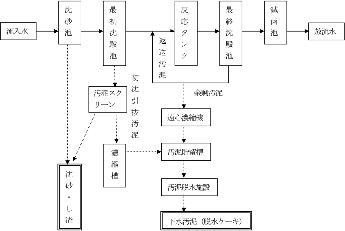
図1 天応浄化センターでの工程
