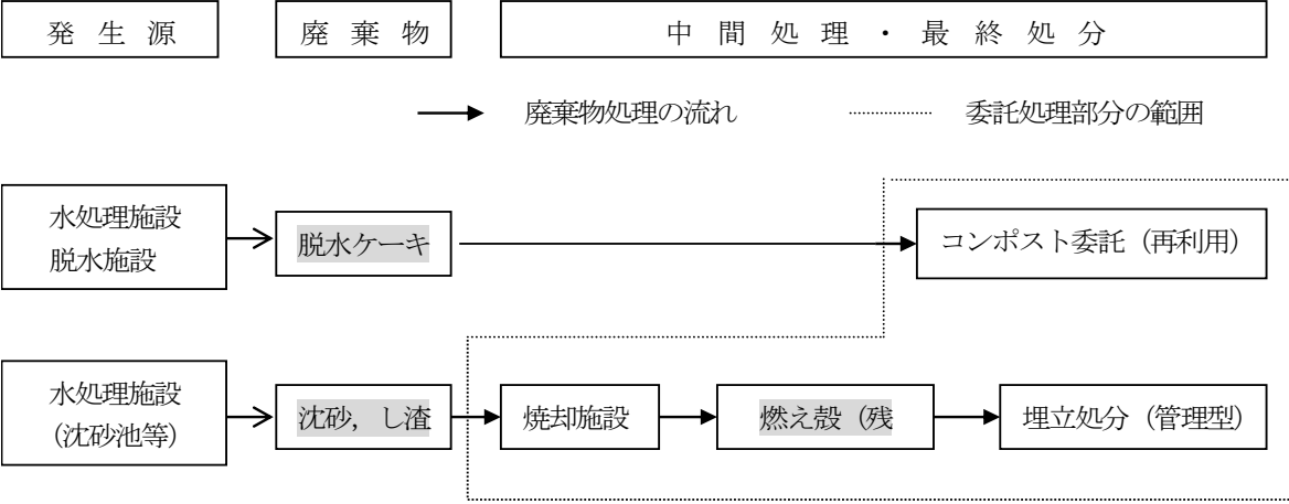
図2 処理の工程
