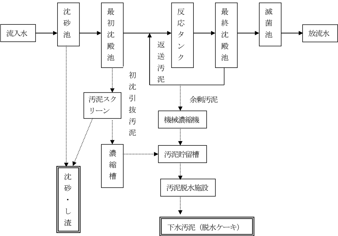
図1 新宮浄化センターでの工程
