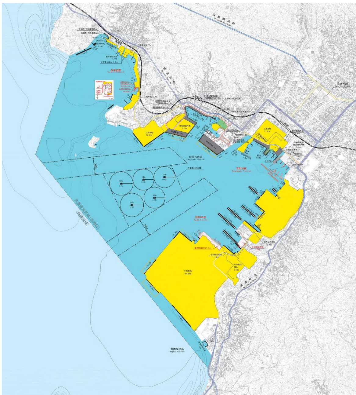
図 1.7 港湾計画図（令和 7（2025）年 10 月作成）【呉港区の拡大図】
