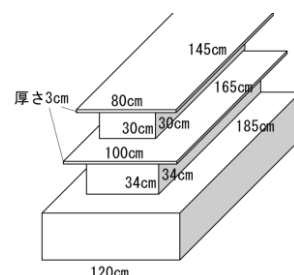
棚の寸法
