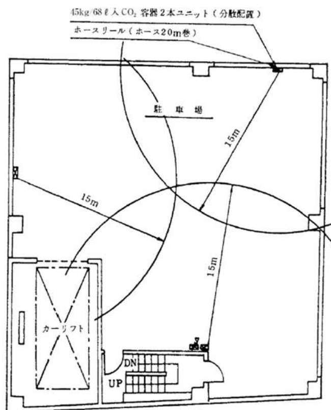
図6-5 二酸化炭素を放出する不活性ガス消火設備移動式図例
