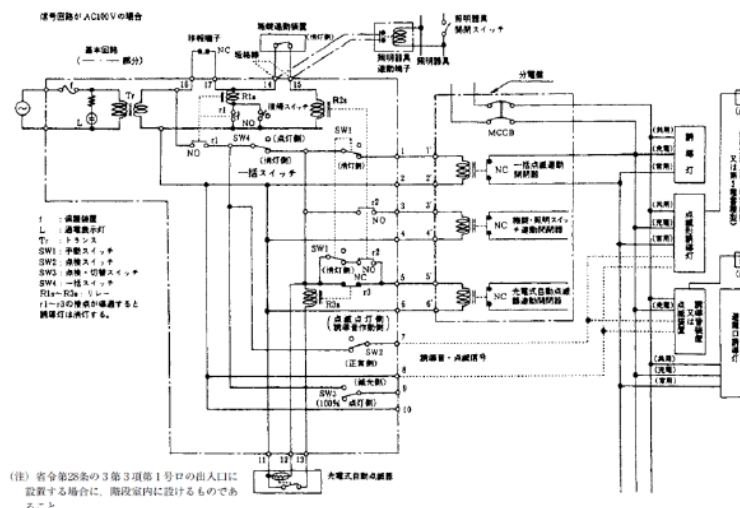
圖16-22 機器結線圖
