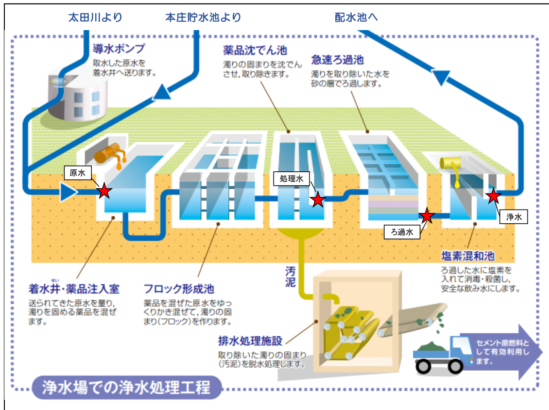
（図4） 浄水場の概略図と検査地点
