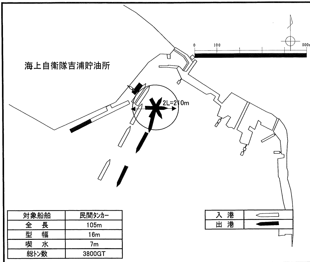
図2-4 第2棧橋操船例図
