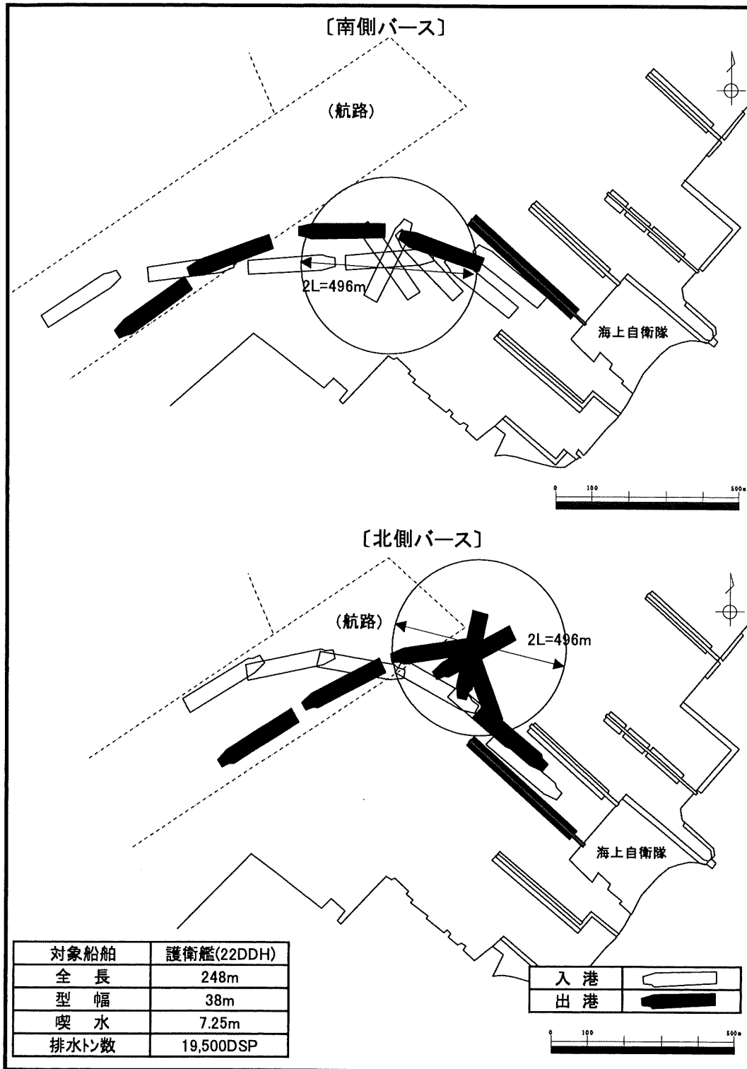
図2-3 Fバース操船例図
