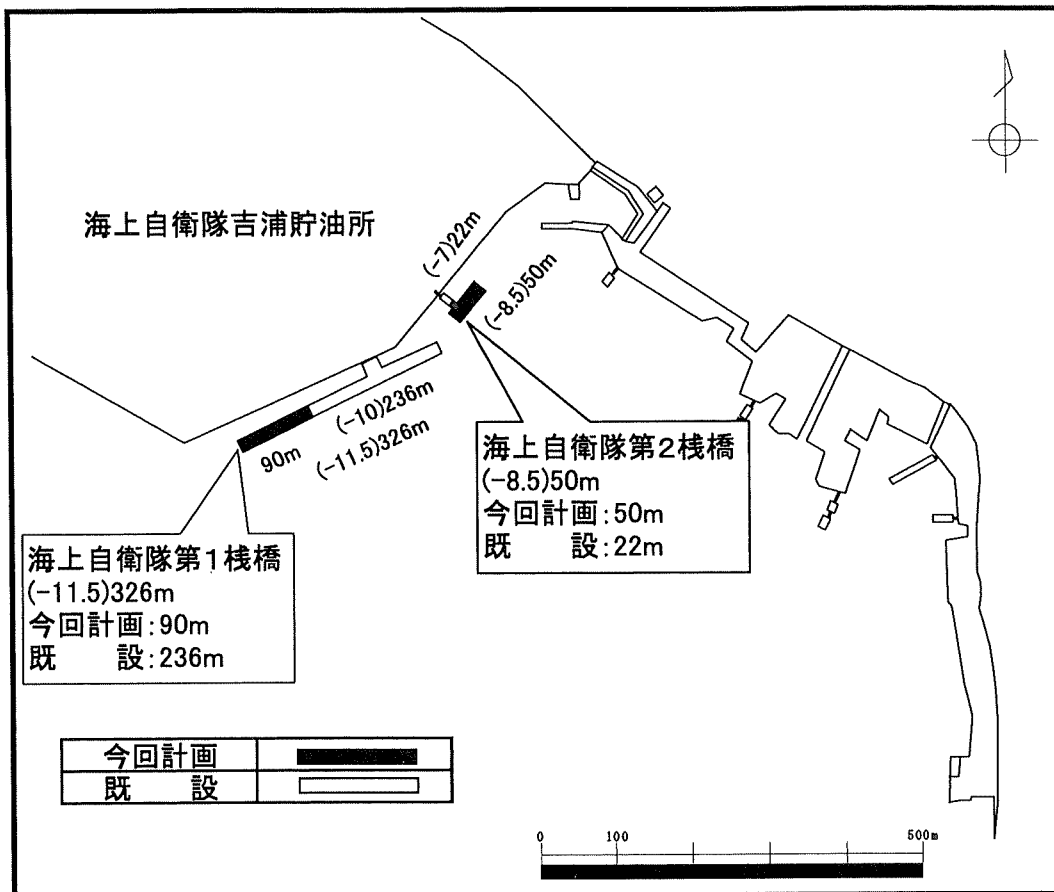
図2-2 専用埠頭計画の位置図(吉浦地区)
