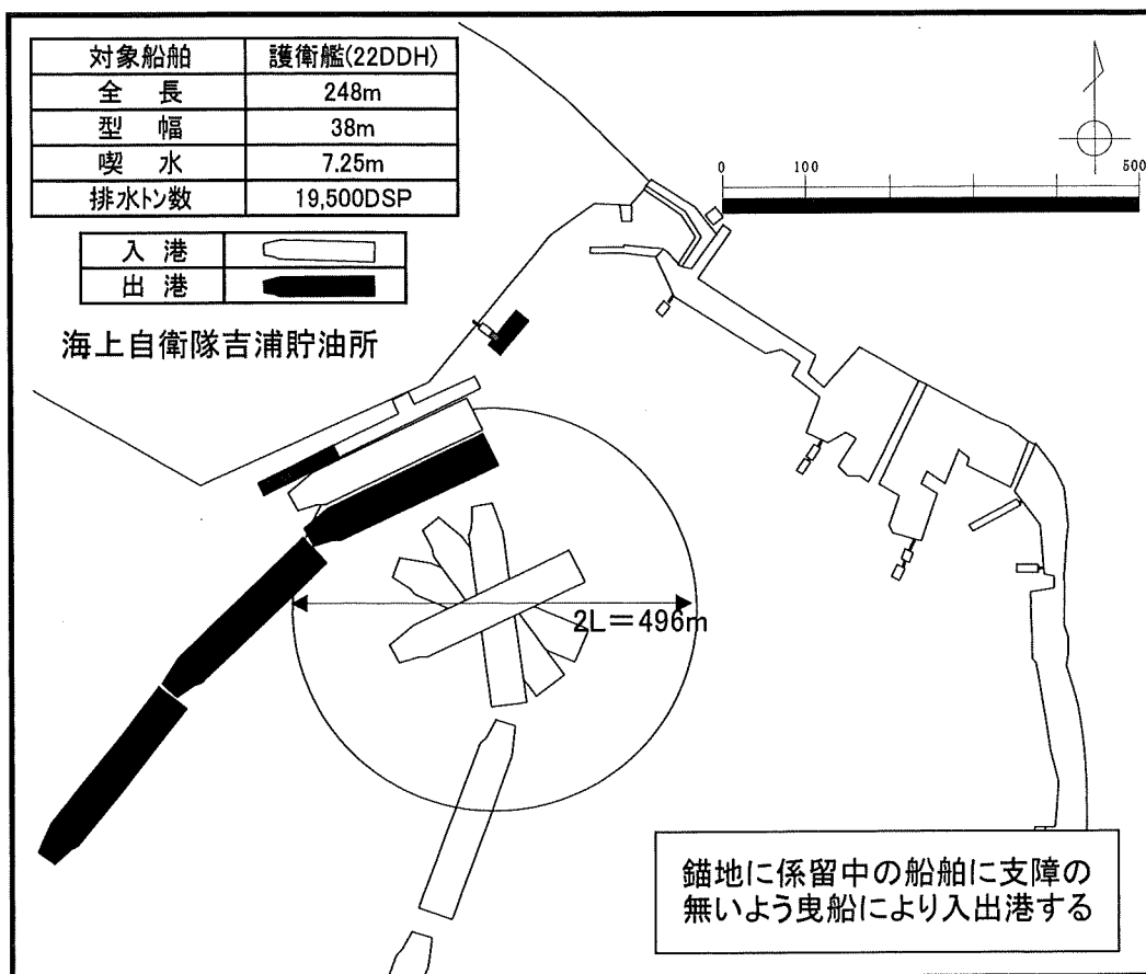
図2-5 第1棧橋操船例図
