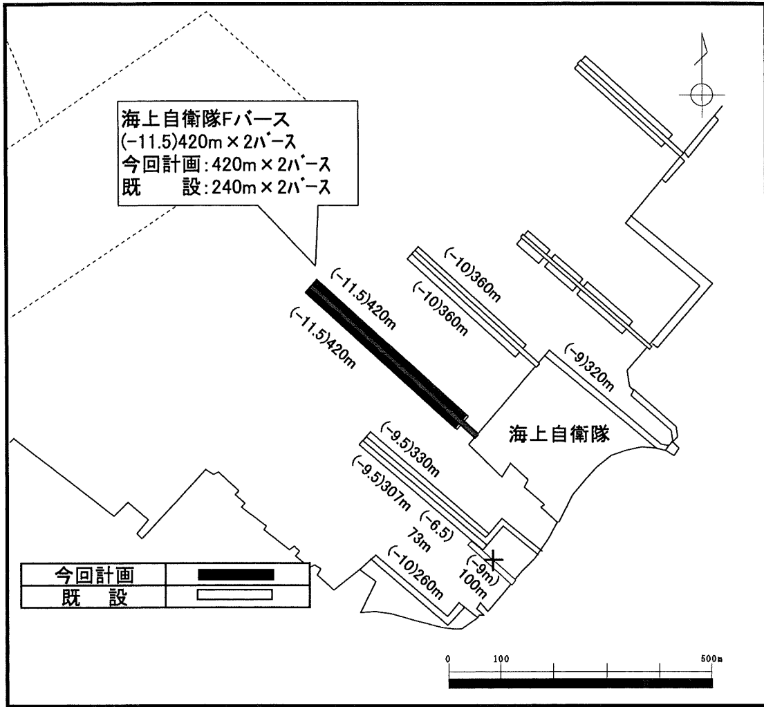
図2-1 専用埠頭計画の位置図(昭和地区)
