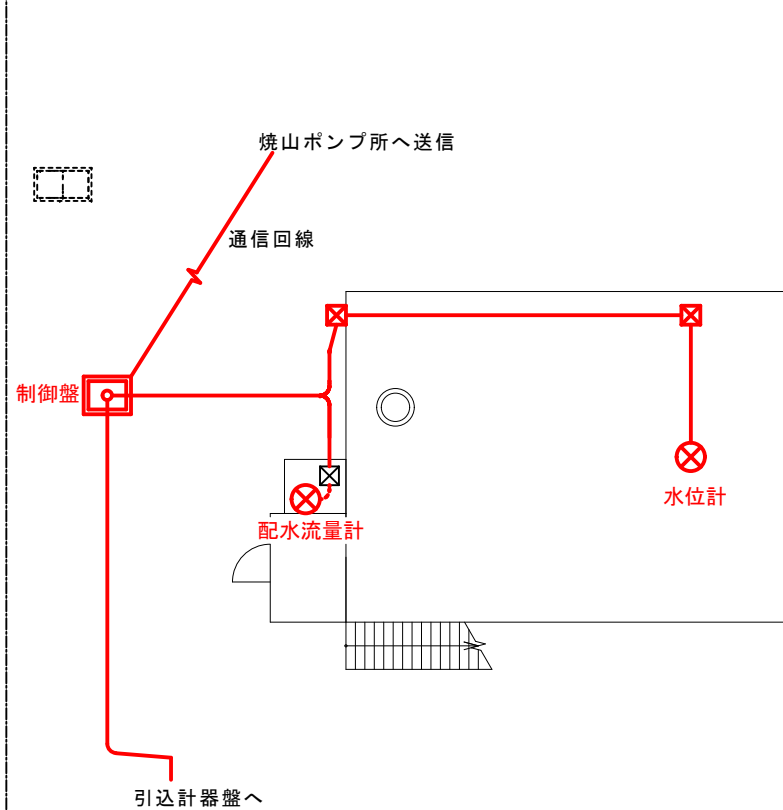
焼山南部配水池平面図
