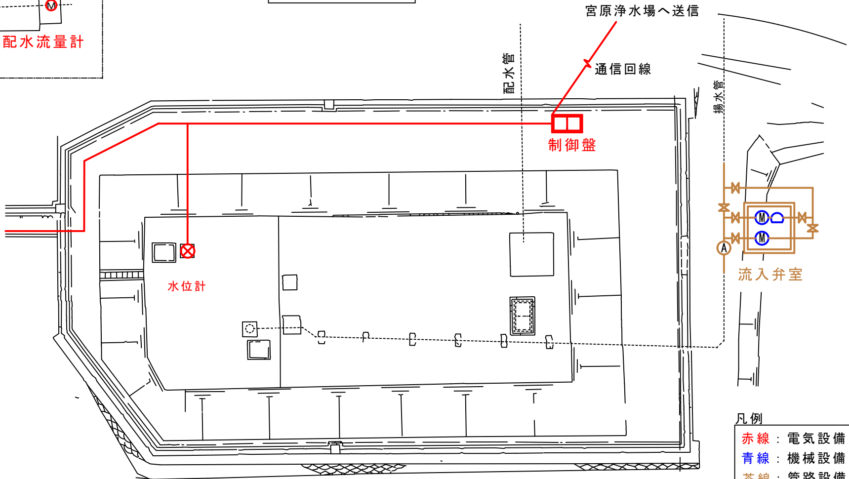
焼山東部配水池平面図
