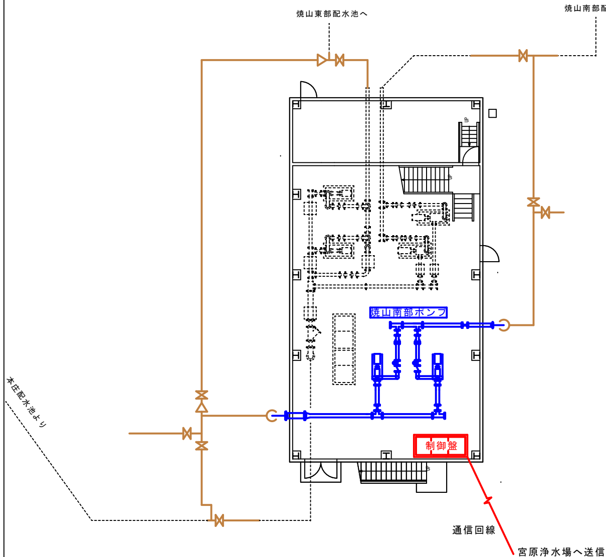
焼山ポンプ所平面図
