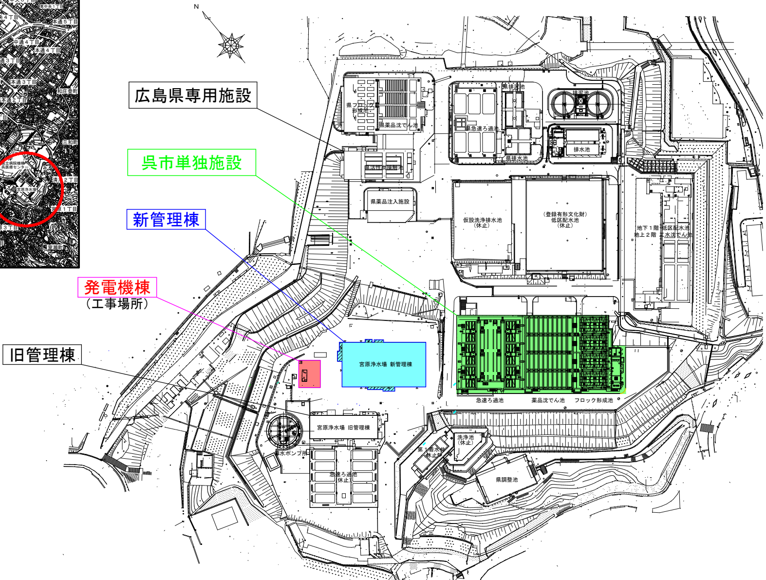
宮原浄水場内平面図
