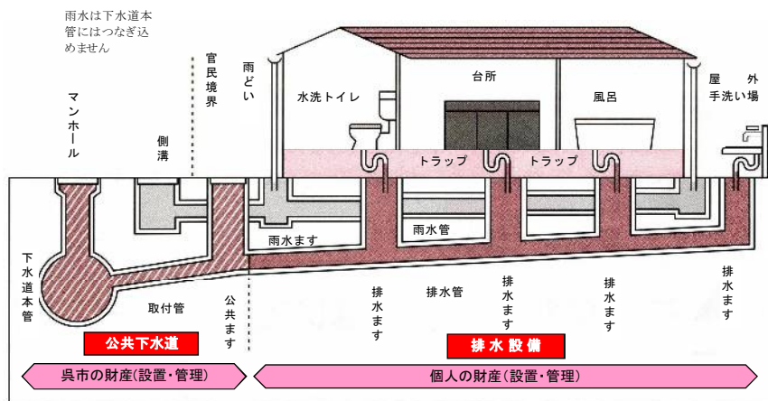
■排水設備維持管理区分表
