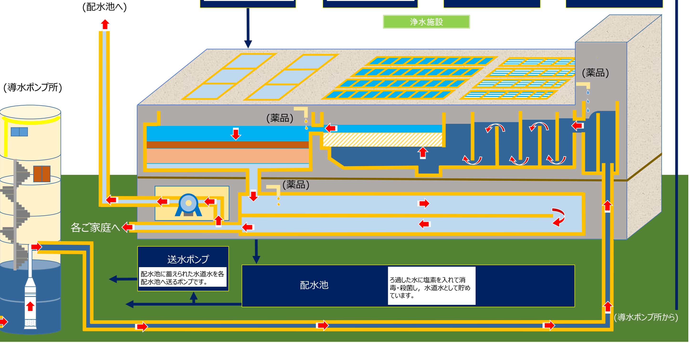
送水施設 配水施設
