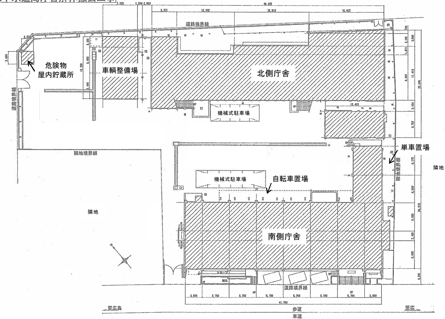
配置図
