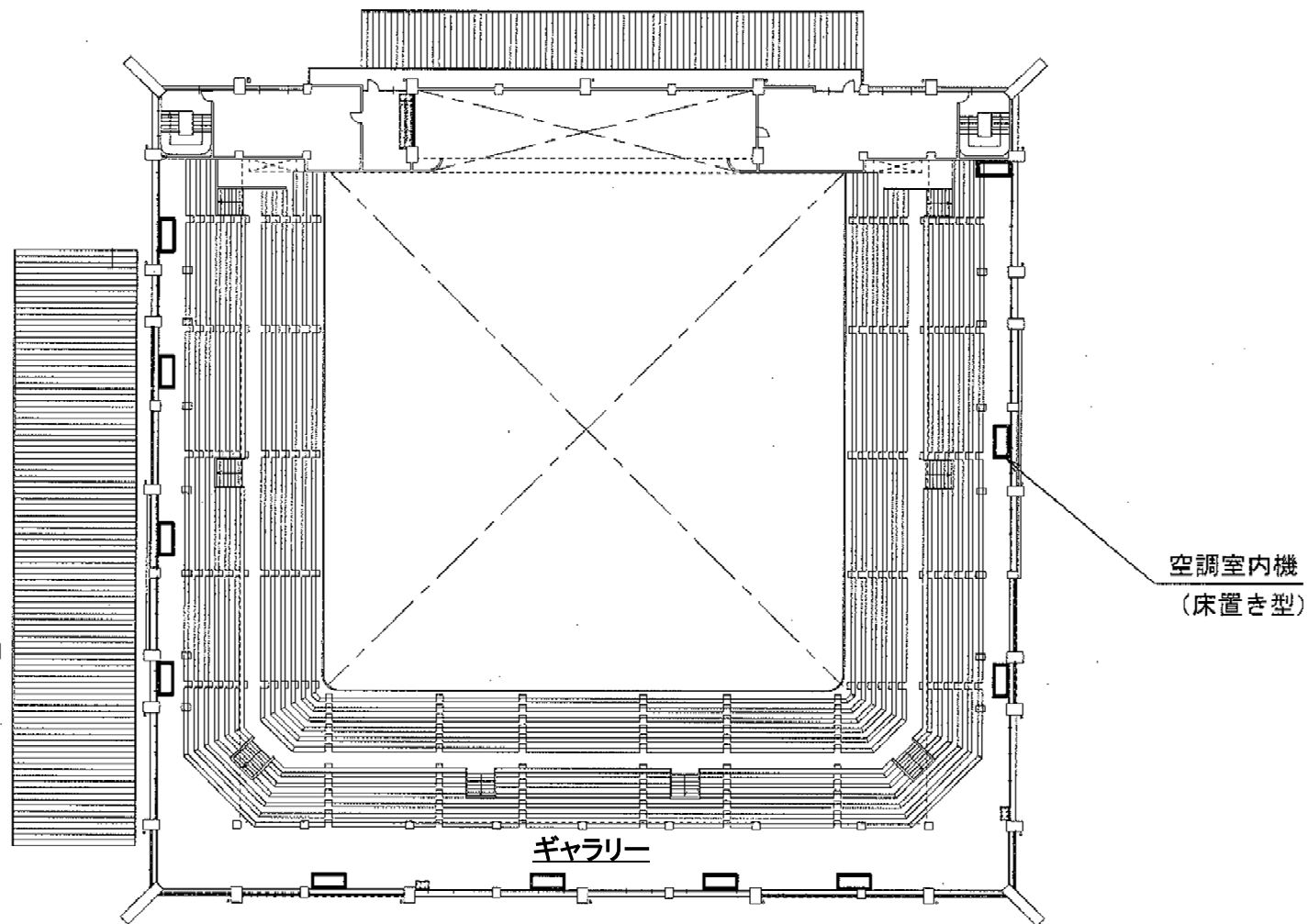
3階平面図
