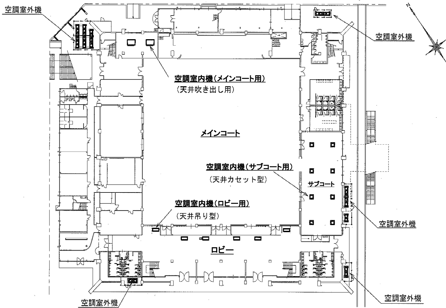
1階平面図
