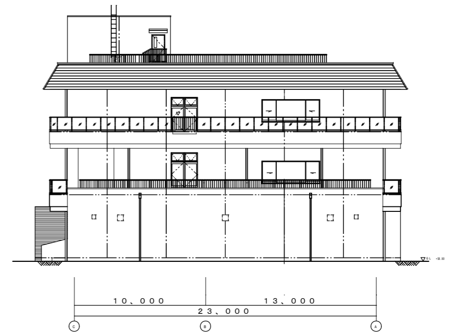
東立面图
