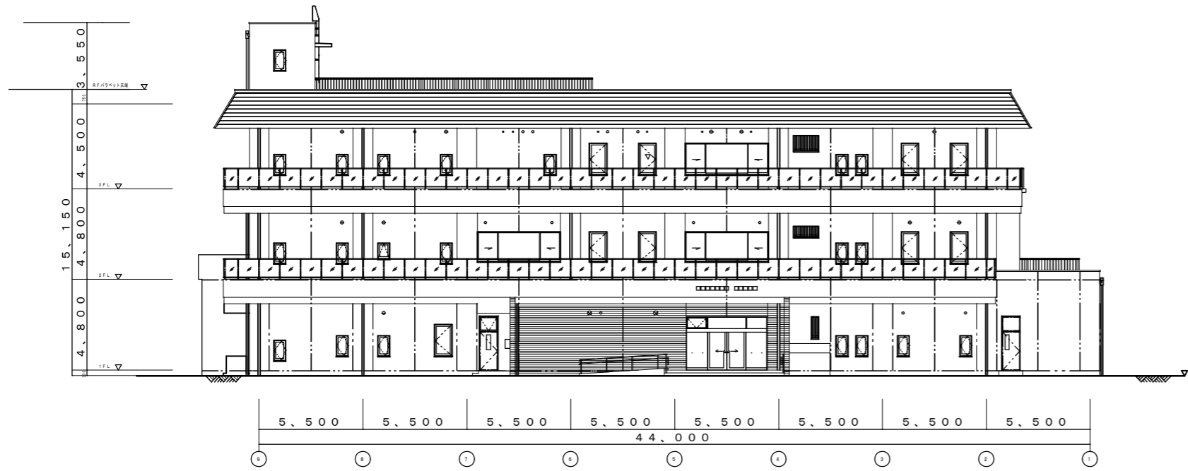
南立面图
