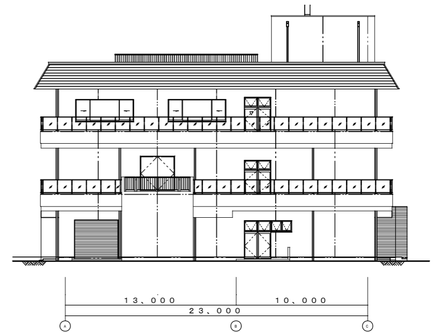
西立面图
