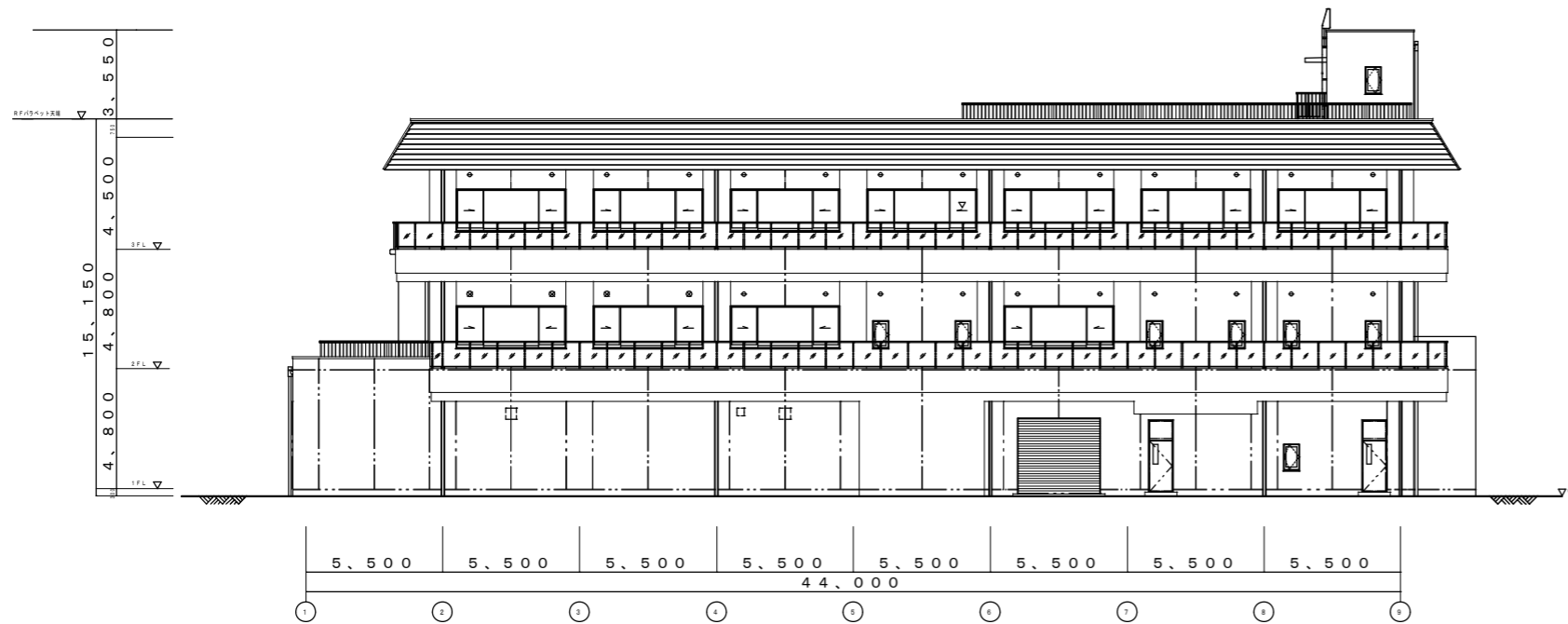
北立面图
